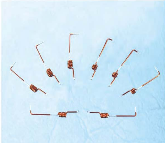
限波弹簧/漆铜线弹簧
