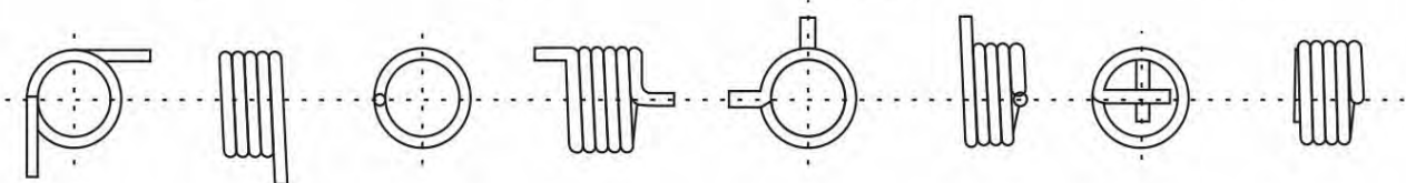
切向脚
